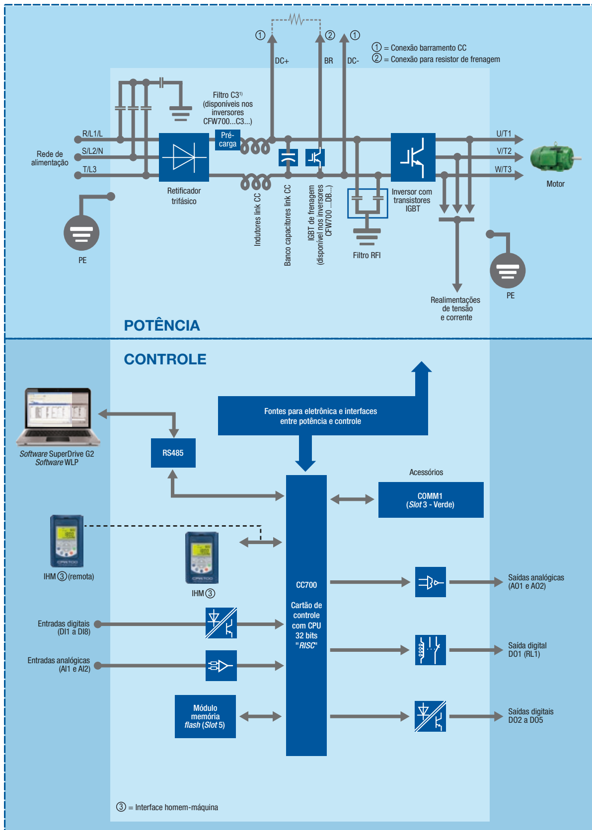
Blocodiagrama do CFW700
